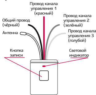
Рисунок 1 - Элементы пульта
