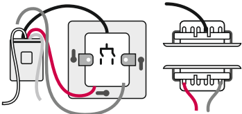
Рисунок 2 - Подключение пульта
