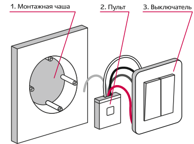
Рисунок 3 - Установка пульта
